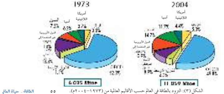
الشكل (٣): التزود بالطاقة في العالم حسب الأقاليم العالمية من (١٩٧٣-٢٠٠٤م).
